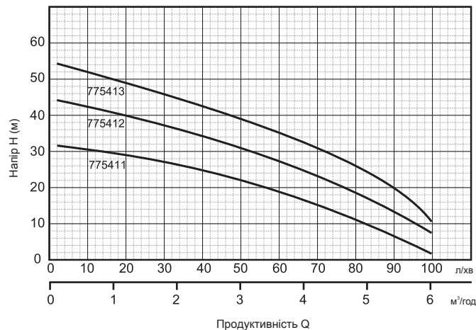
Мал. 2. Діаграми продуктивності відцентрових багатоступеневих насосів.
