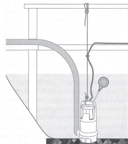
Рис. 1. Схема дренажной системы.
