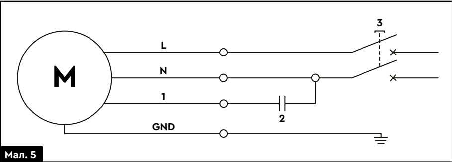
Схема підключення насоса (мал. 5)
